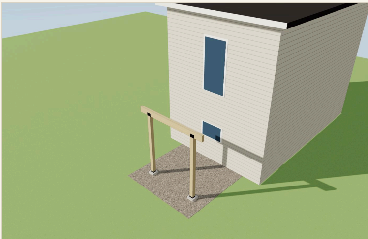
Step 4 · Beams — DROP 4x10 DF (2 posts)
